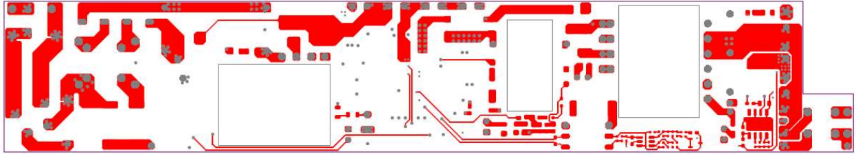
Top layer
