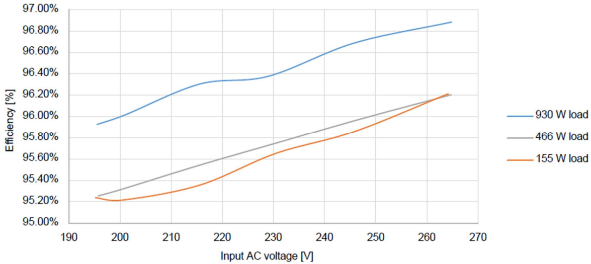
PFC Stage 效率曲線(不同負載及輸入電壓條件下)
