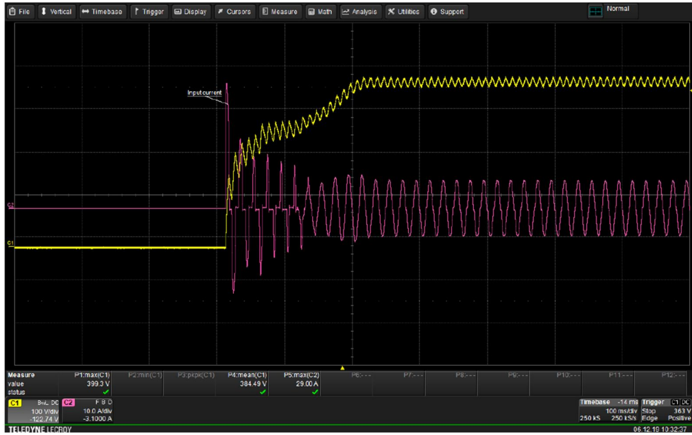
930W 之負載條件下啟動波形(C1:輸出電壓,C2:輸入電流)
