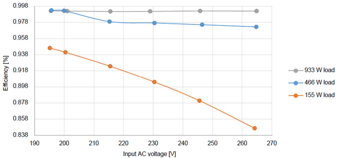
PFC Stage 功率因數曲線(不同負載及輸入電壓條件下)
